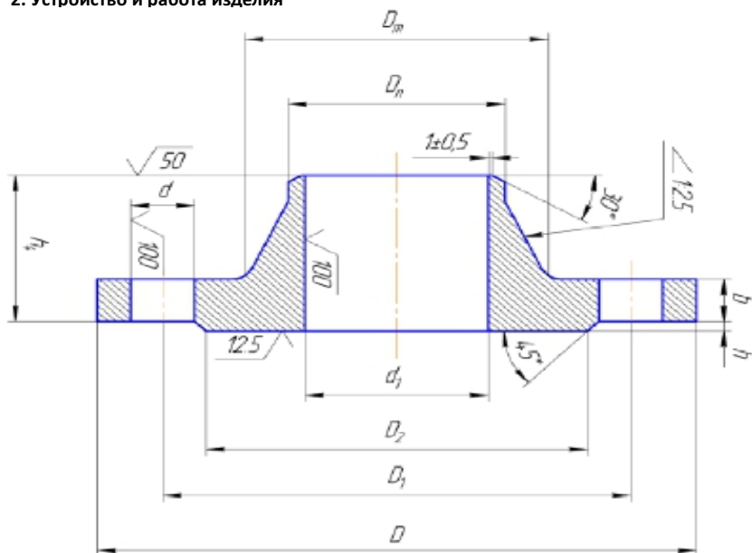
Табл.1 Размеры Фланцы: AISI304 Дn15-150 Pn16; AISI316 Дn15-150 Pn16; 12X18H10T Дn15-150 Pn16.
